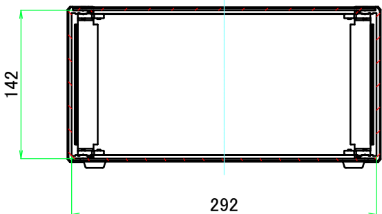
B-B ( 1 : 5 )
