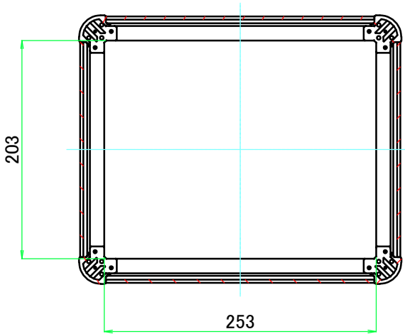
C-C ( 1 : 5 )
